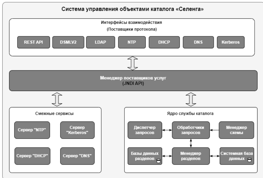
Структурная схема Системы управления объектами каталога «Селенга» Рисунок 1
